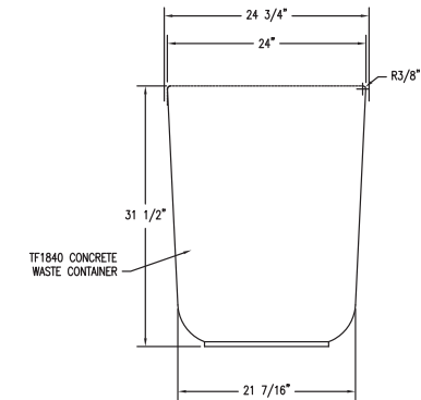
2 ELEVATION VIEW Scale: 1/8" = 1"
