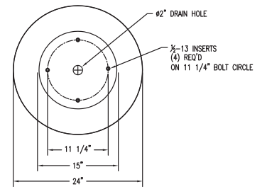
3 BOTTOM VIEW Scale: 1/8" = 1"
